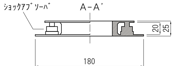
A-A' 車載用振動吸収ベース
